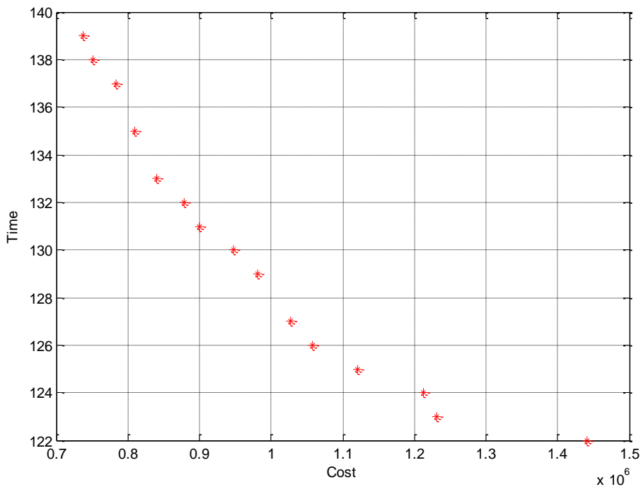
شکل ۸ - نمودار مجموعه جواب نا مغلوب در الگوریتم MOPSO
