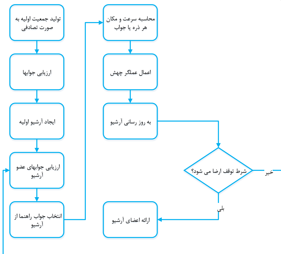
شکل ۶ - فلوجارت الگوریتم MOSPO
